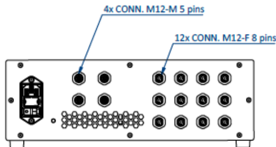
12xUV 照射器のための電源
